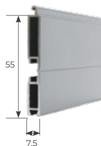
STANDARD Terminale 7x55 in alluminio estruso
