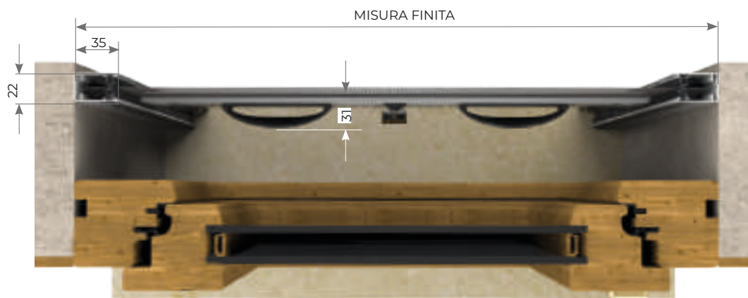
VARIANTE A RICHIESTA AGGANCIAMENTO PIATTO
