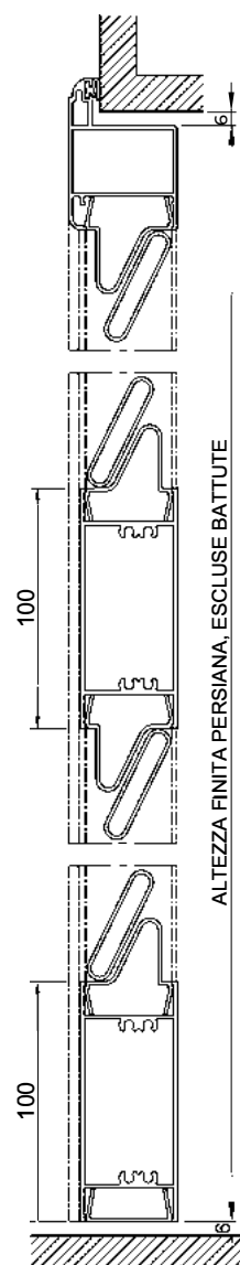
SEZ. VERTICALE PORTAFINESTRA
