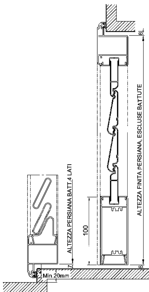
SEZ. VERTICALE FINESTRA
