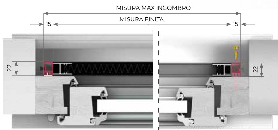
SEZ. ORIZZONTALE FISSAGGIO CON CLIP
