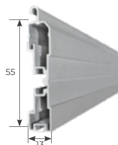
STANDARD Terminale 13x55 in alluminio estruso
