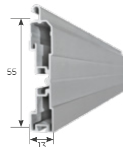
STANDARD Terminale 13x55 in alluminio estruso
