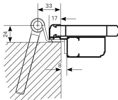
CARDINE A MURO
