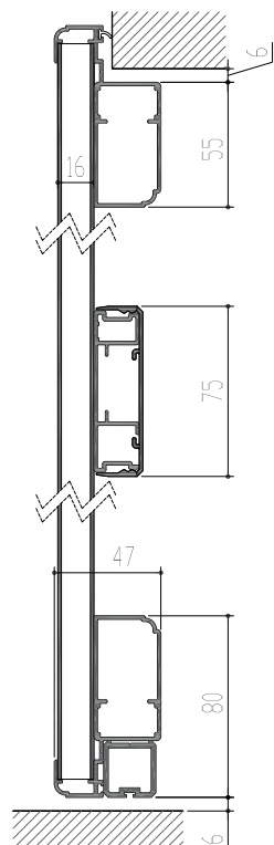
CARDINE A MURO
