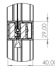
DETTAGLIO U SCALA 1 : 2
