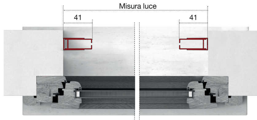
SEZ. ORIZZONTALE
