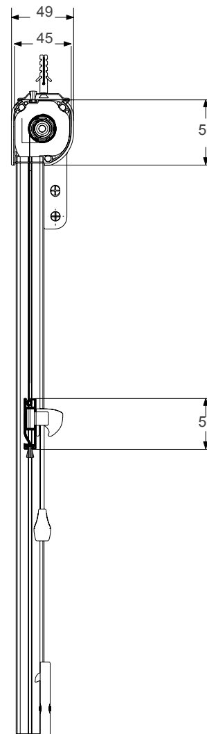
SEZIONE VERTICALE
