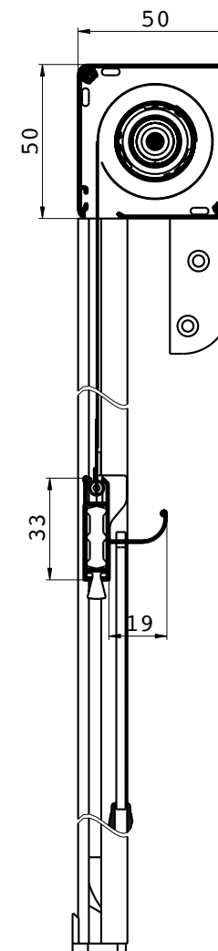
SEZIONE VERTICALE
