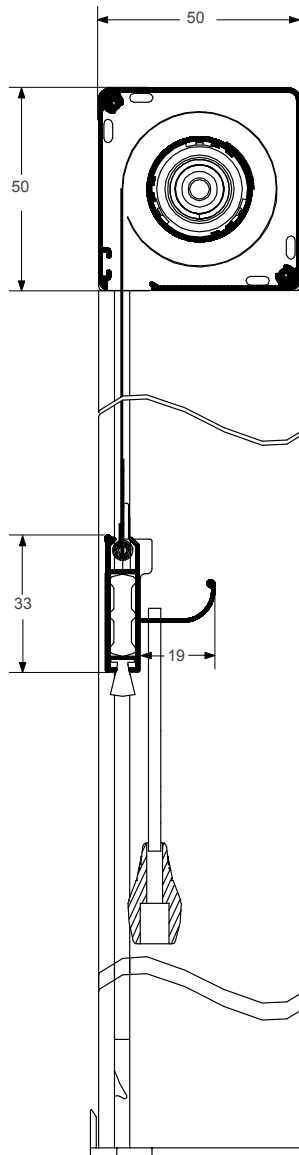
SEZ. VERTICALE
