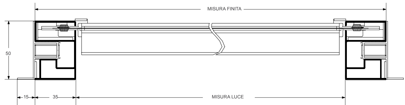
SEZ. ORIZZONTALE
