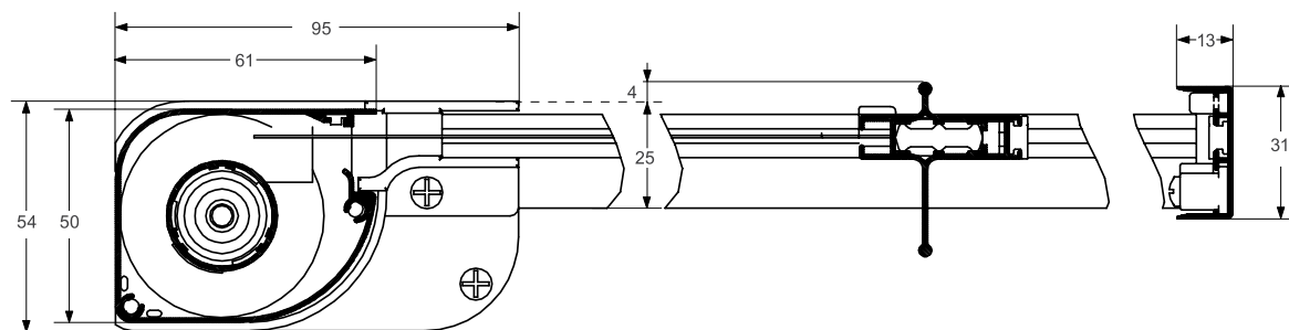
SEZIONE ORIZZONTALE
