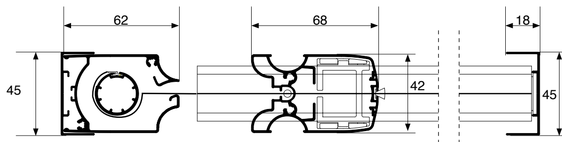
SEZIONE ORIZZONTALE
