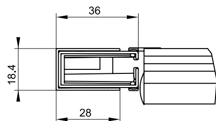
PARTICOLARE "B"
