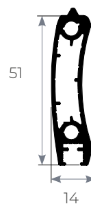
PROFILO LAMELLA
