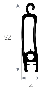
STECCA SUPERIORE
